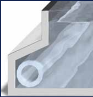
Unterflur – tiefliegender Rucksackschacht Verlängerung am Beckenboden
