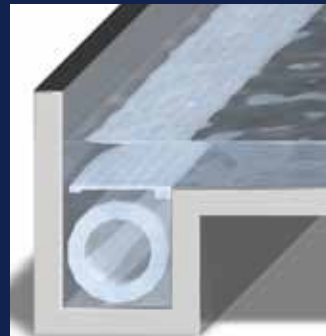
Unterflur – Schacht im Beckenboden
